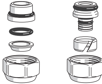
Conectori eurokonus (livrați separat)
